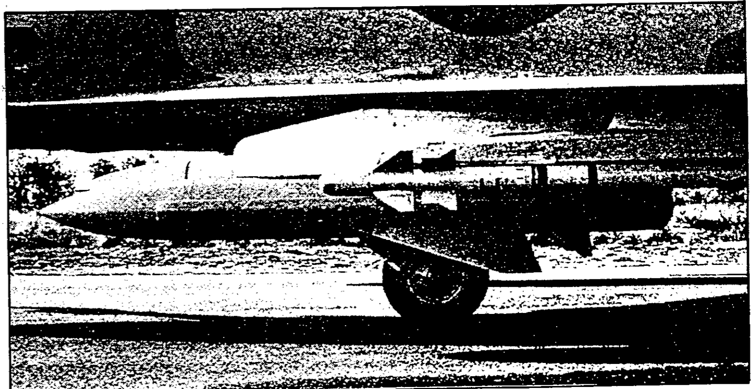
الصواريخ الفرنسي الموجه على الاشعة الرادارية «ارمات» مع الصواريخ «ماجيك» جو-جو
